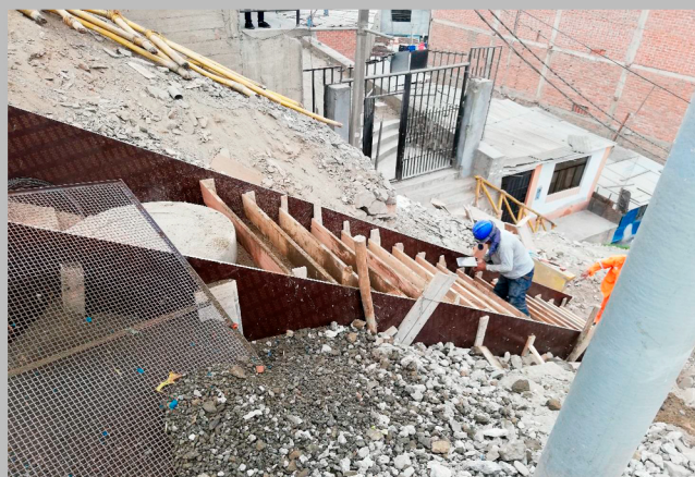
CONSTRUCCIÓN DE ESCALERAS REPLANTEADAS LLENADO
