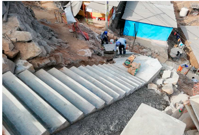
CONSTRUCCIÓN DE GRADERIA TRAMO 2 RAP 01
