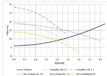
CURVA SISTEMA / RENDIMIENTO DE BOMBA
