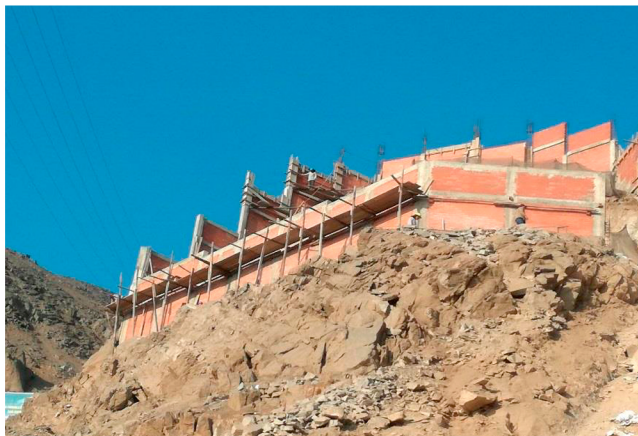
CONSTRUCCIÓN DE CERCO PERIMÉTRICO RAP 01
